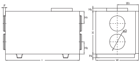
HRS-EH/HRS-WH 700-1900
