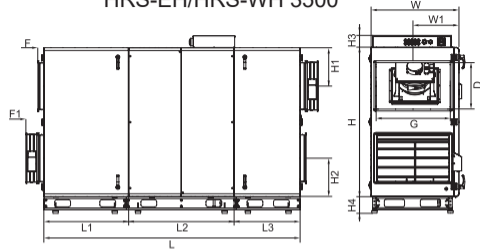
HRS-EH/HRS-WH 3500
