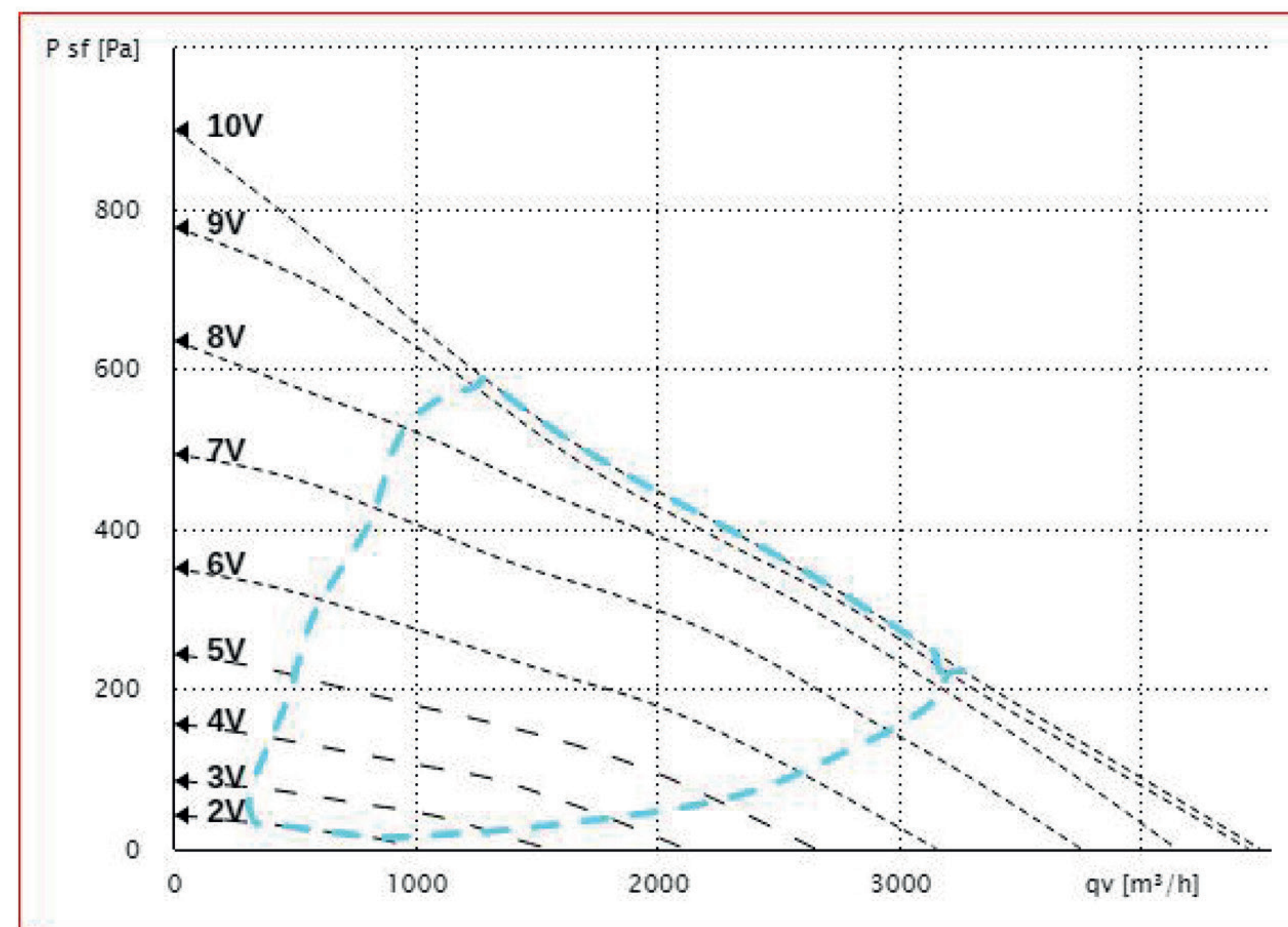
BFA 500 EC K 01
