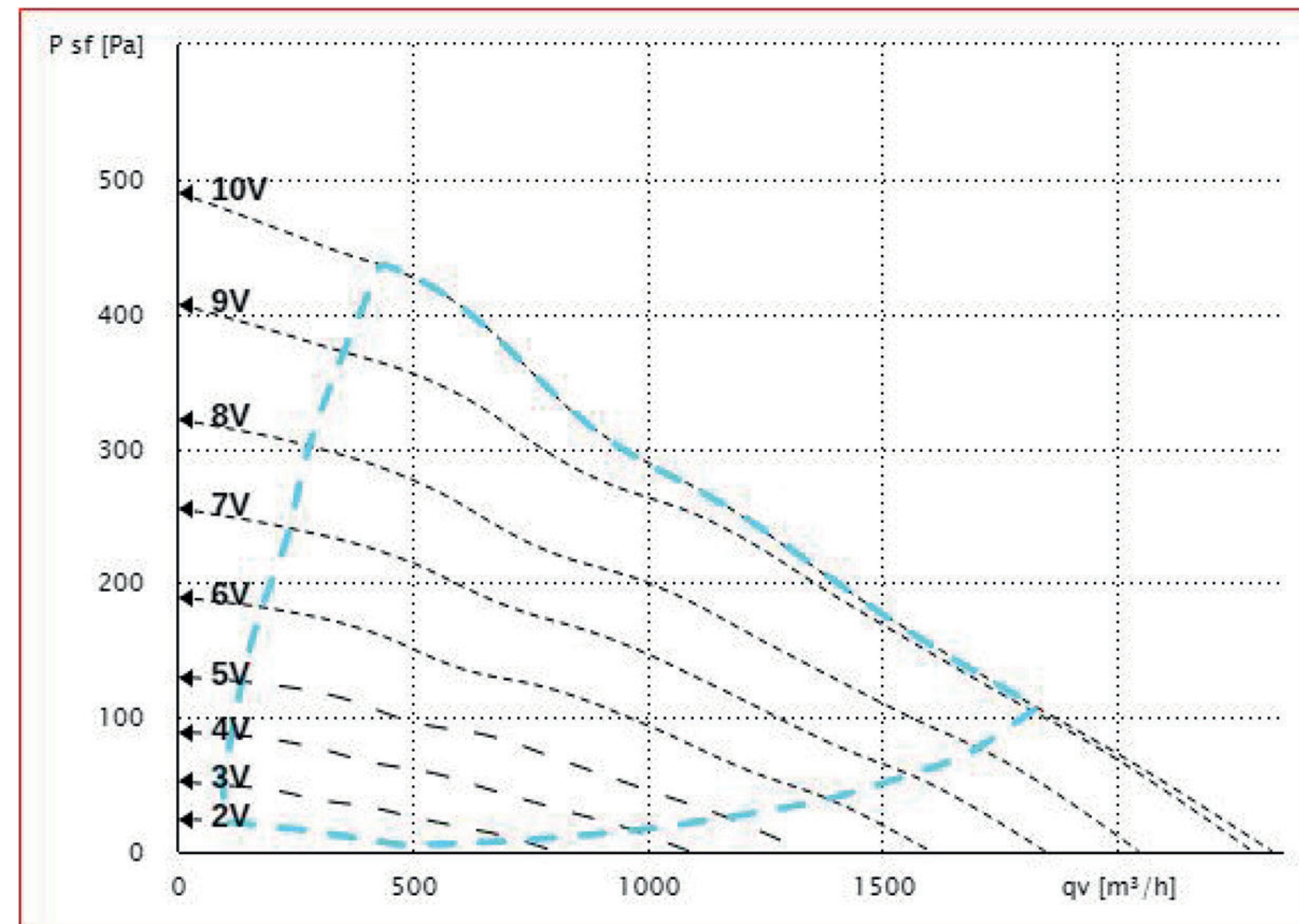
BFA 400 EC K 01
