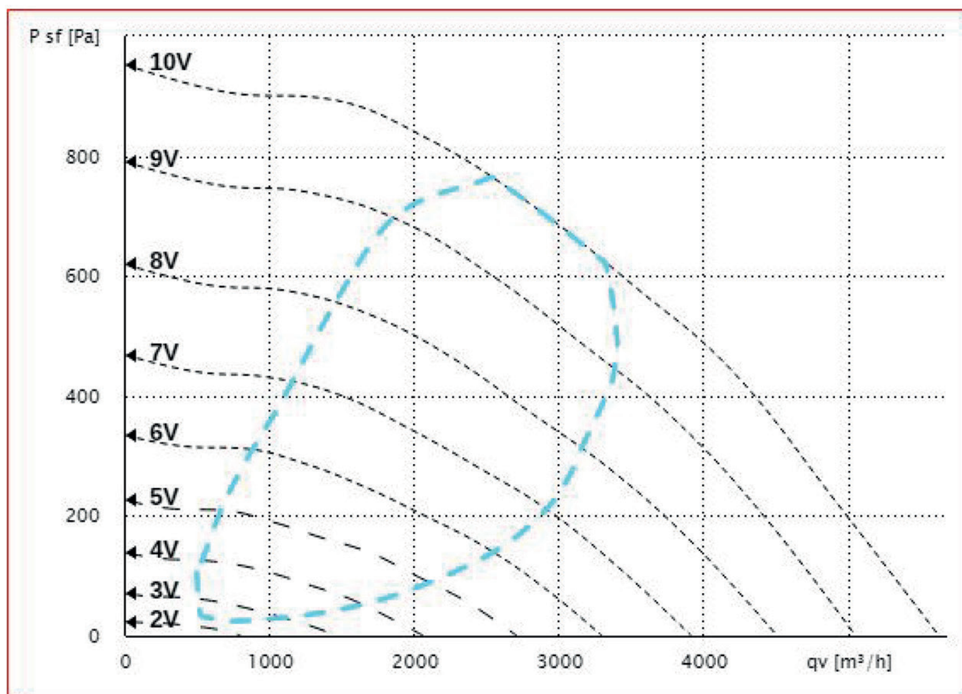
BFA 450 EC K 01
