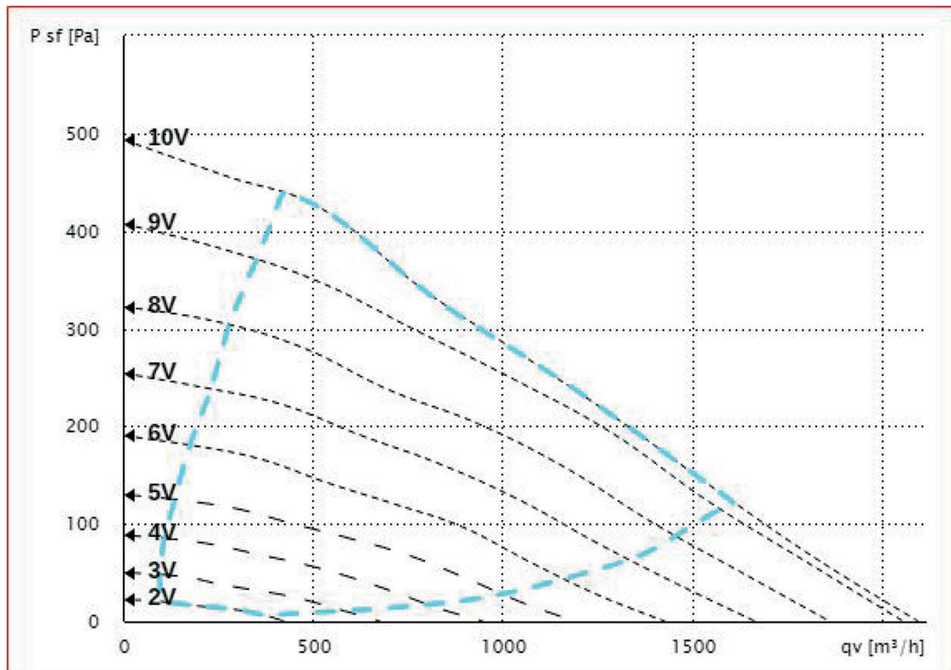
BFA 355 EC K 01
