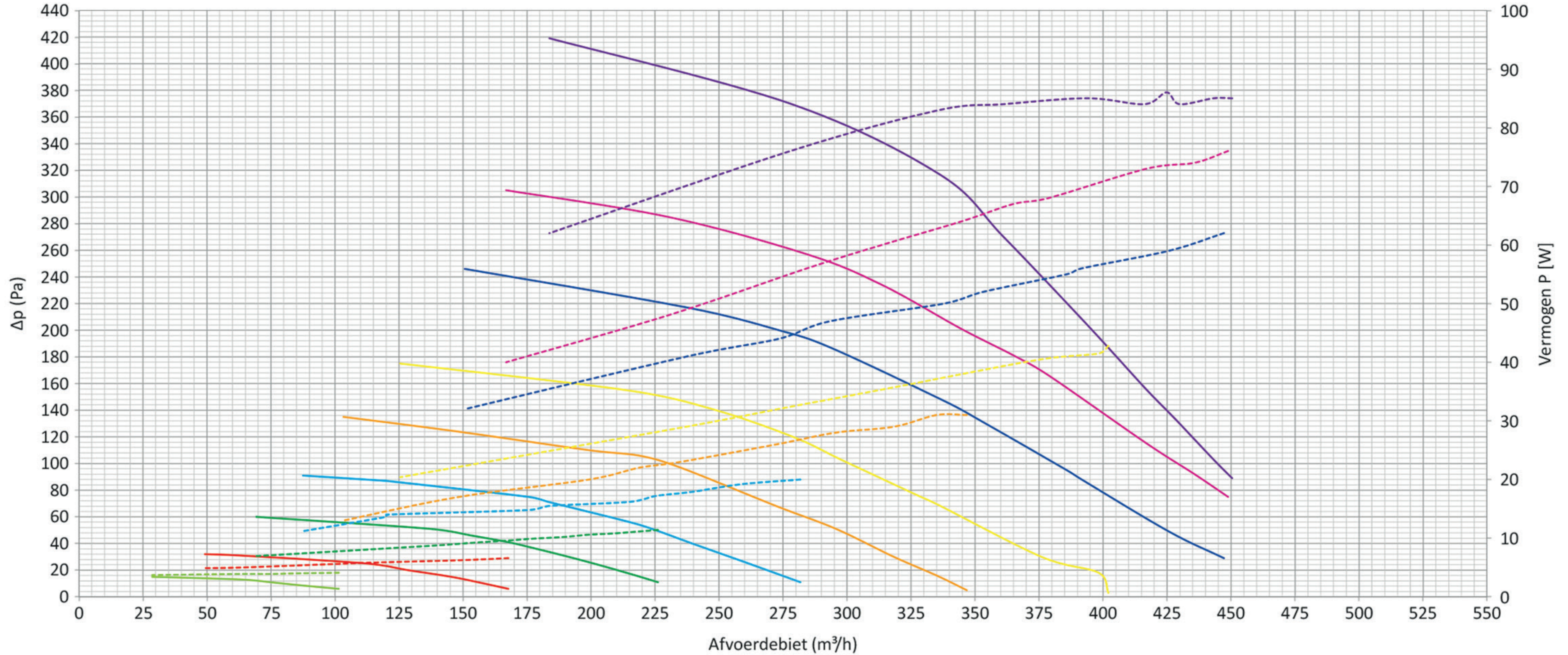
Ventilatorcurve's R3G140-AF17-12 druk en vermogen i.f.v. debiet
