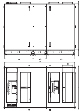
HRS-REV/HRS-RWV 5500
