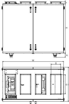
HRS-REV/HRS-RWV 2500
