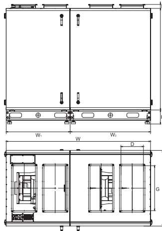
HRS-REV/HRS-RWV 3500
