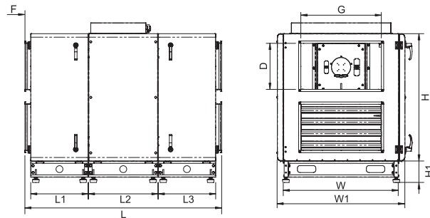
HRS-REH/HRS-RWH 2500-5500
