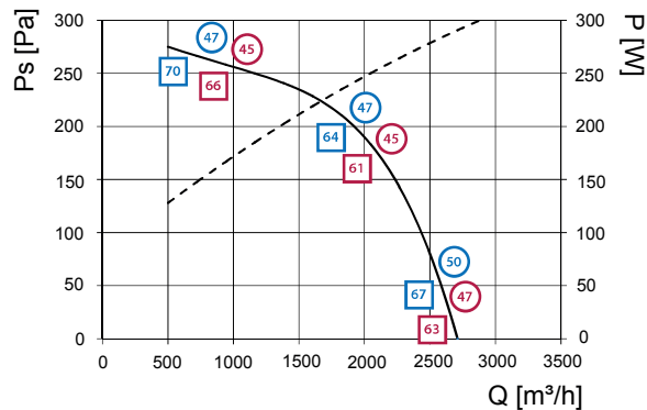
BFSA-I 355
