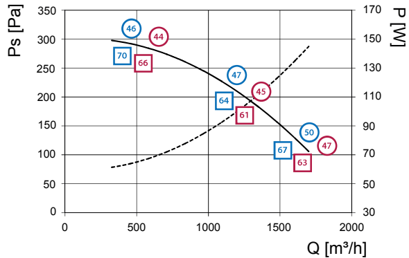
BFSA-I 400
