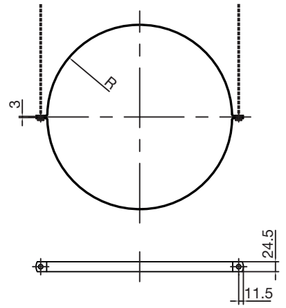
Ø450 - Ø1000
